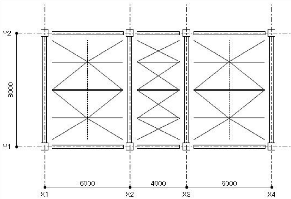
屋根伏図
