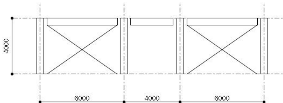
Y1、Y2通り 軸組図
