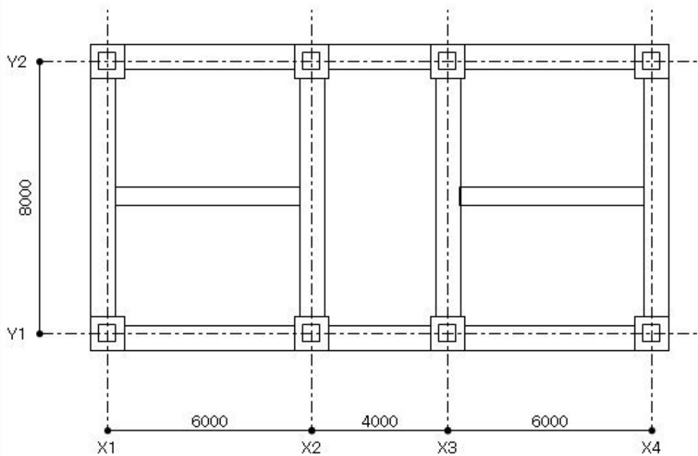
1階床伏図
